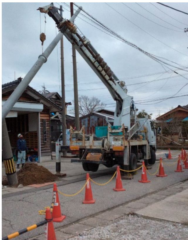
配電設備復旧作業の様子
